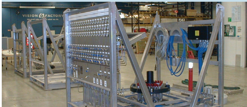
SCM Test Stand
